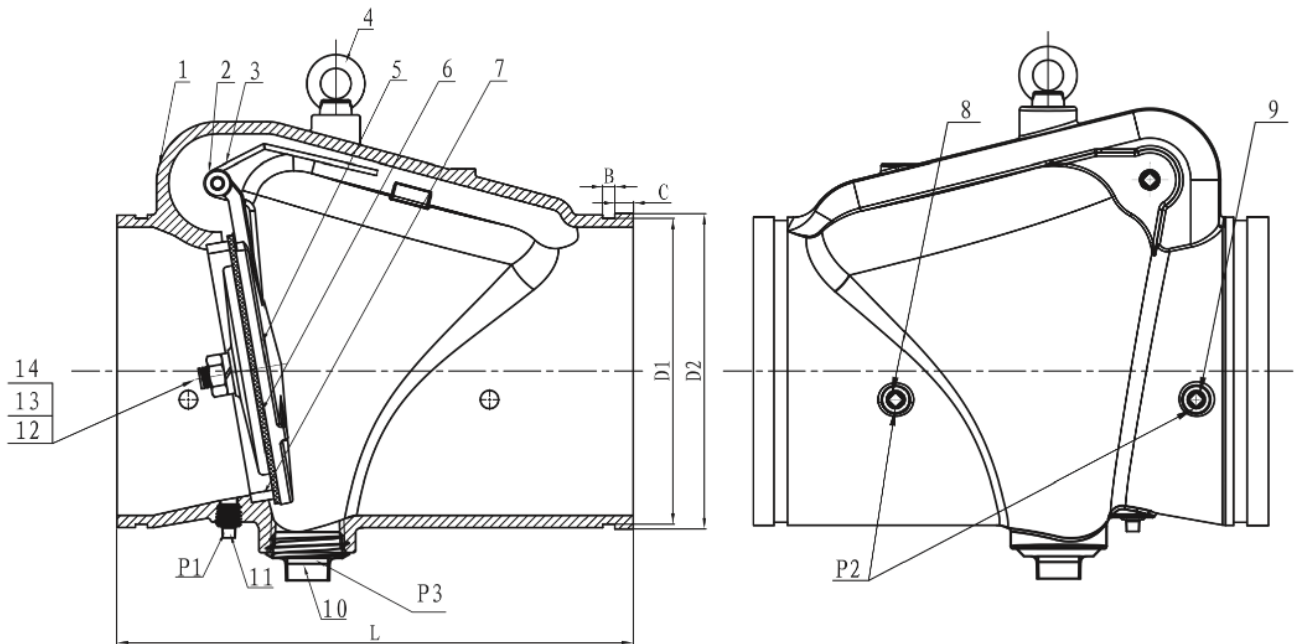
Габаритные размеры
